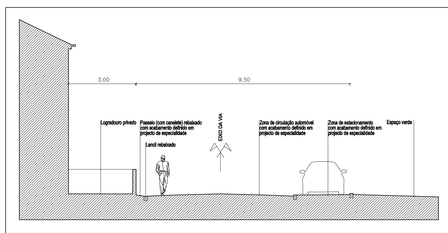
P1. PORMENOR TIPO DOS ARRUIJAMENTOS COM PASSO REBAIXADO e ESTACIONAMENTO - 1 SENTIDO DE TRÁFEGO (ESC. 1:100)
