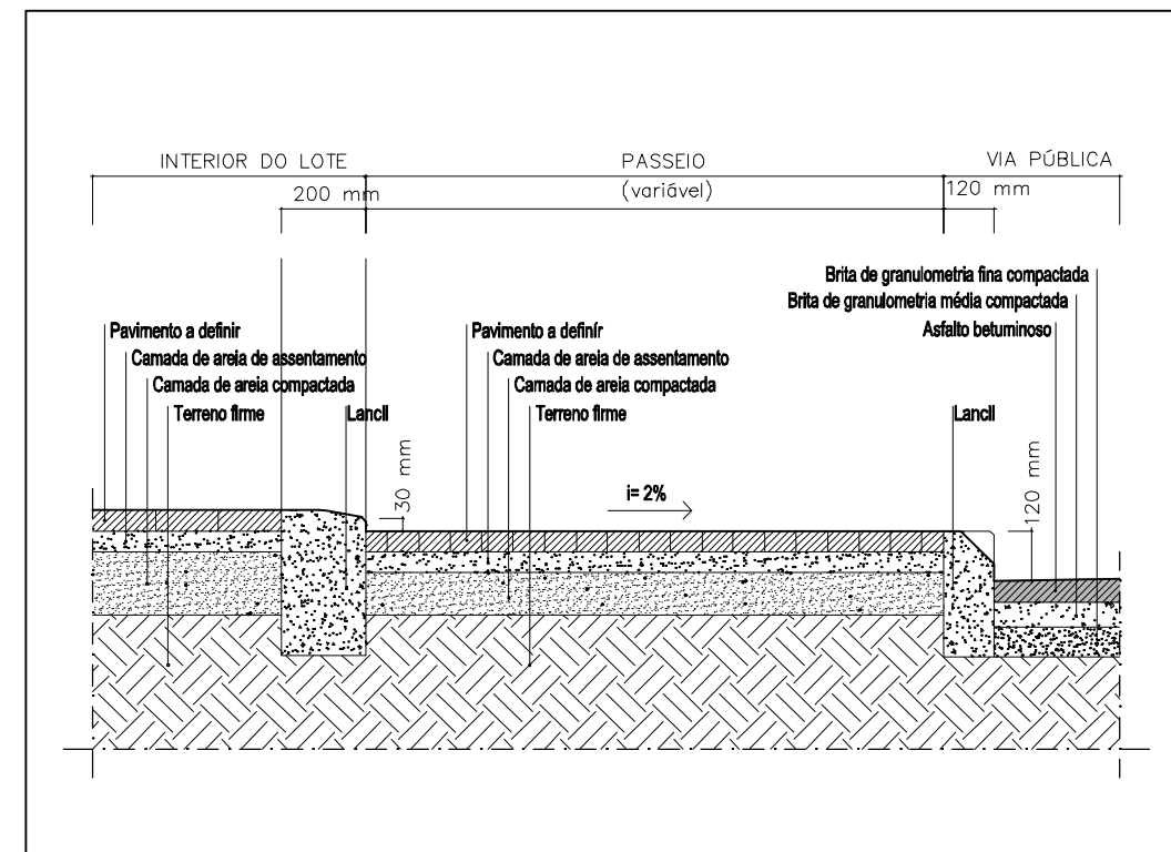
P4. PORMENOR TIPO DO PASSO E LANCIL (ESC. 1:20)
