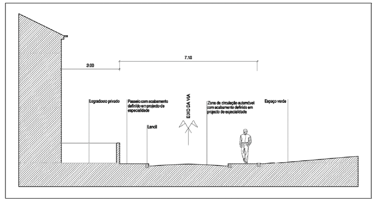
P1. PORMEIOR TIPO DOS ARRUAMENTOS COM PASSEIO - 1 SENTIDO DE TRÁFEGO (ESC. 1:100)
