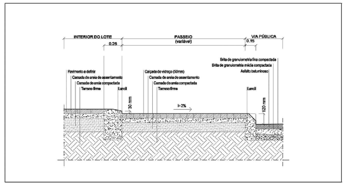
P2. FORMEIRO TIPO DO PASSEIO E LANCIL (ESC. 1:20)
